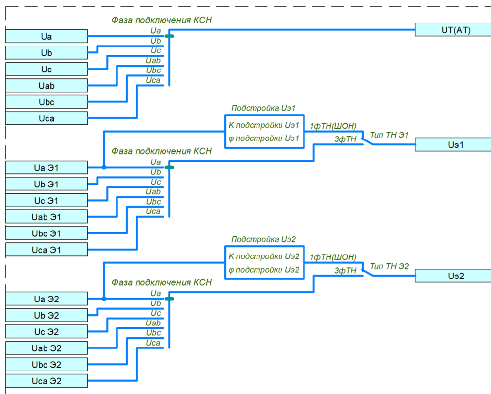
Рисунок 2.13 – Выбор величин напряжений для КСН
