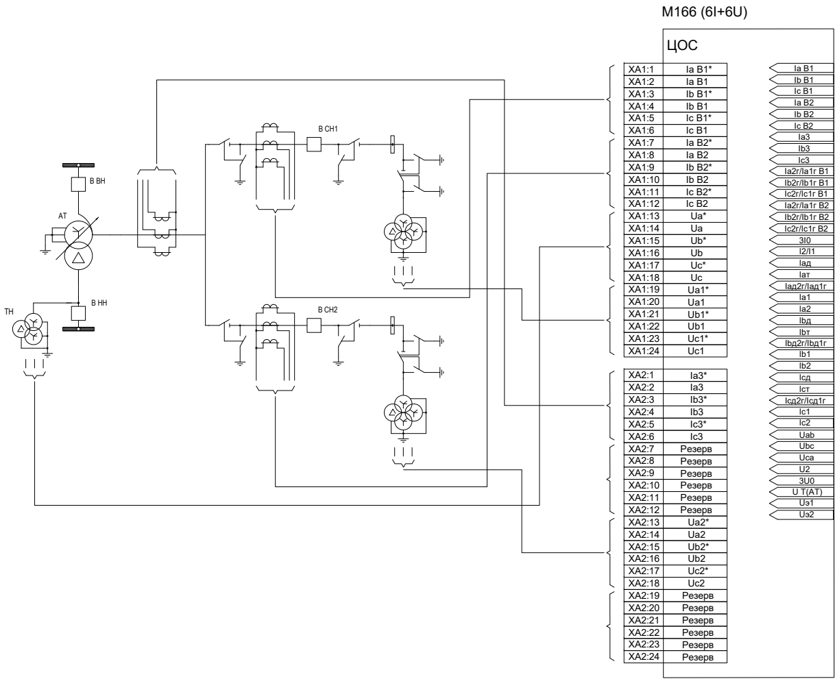
Рисунок Б.1 – Вариант подключения аналоговых цепей ТТ и ТН к устройству
