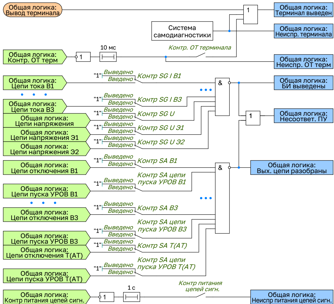
Рисунок 2.30 – Функциональная схема общей логики
